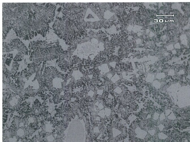
溶着金属組織一例
